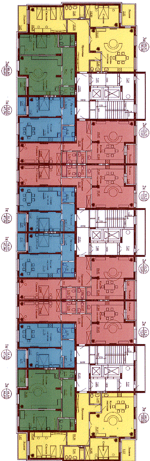
План типового этажа жилого дома для ЖК "Тротон"
